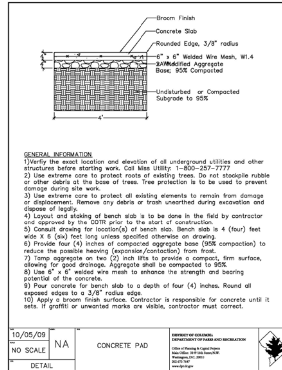
4 CONCRETE PAD DETAIL SCALE: NA
