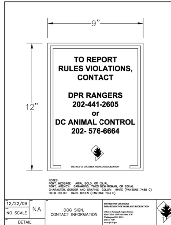
5 DOG PARK SIGNAGE SCALE: NA
